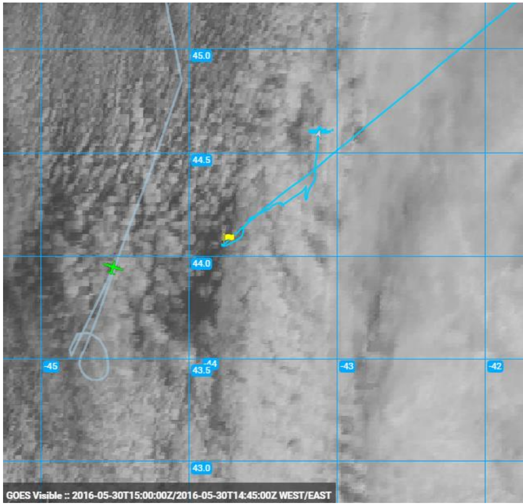
1515Z_LowLevelZPatternLeg
