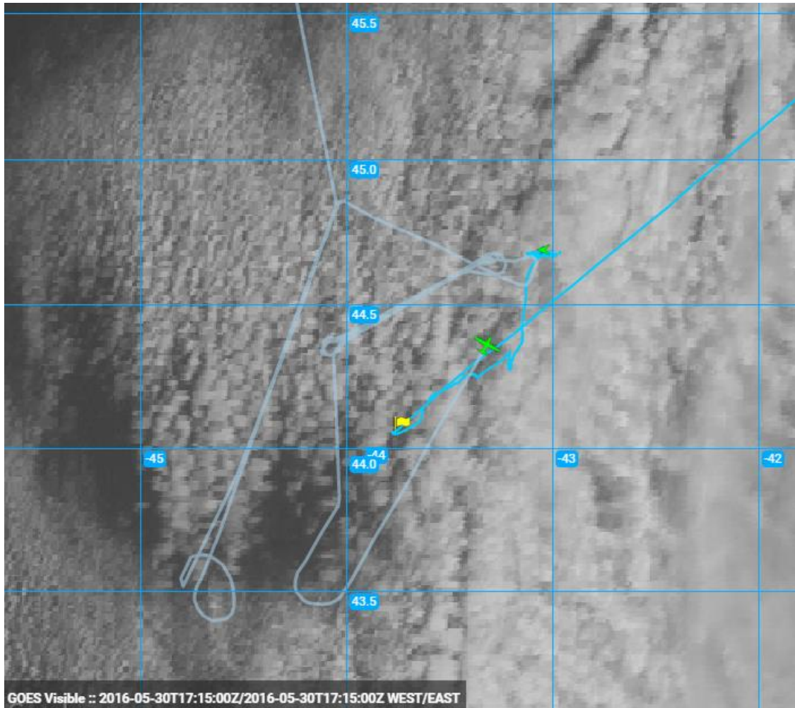
1735Z_HighAltZpattern
