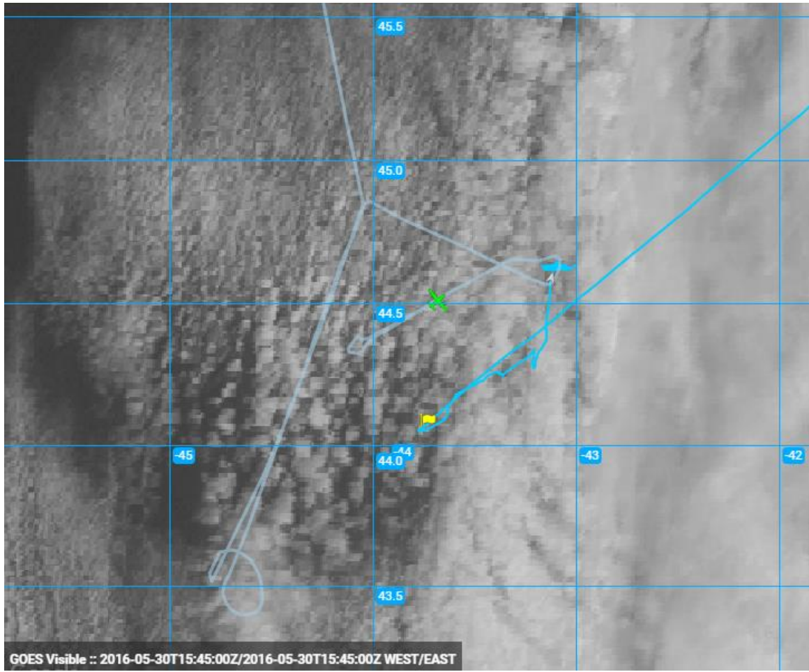
1605Z_CloudModule_BiggerView
