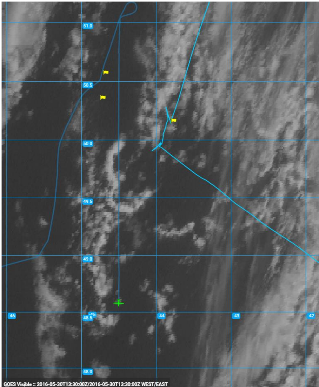
1350Z_HighAlt_N-S_Survey
